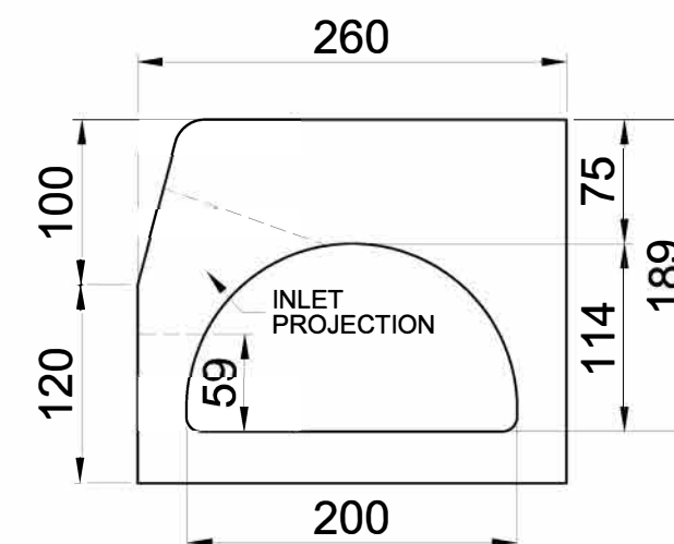
RIGHT ELEVATION
