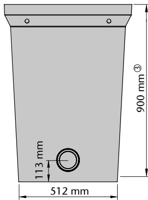
Optional riser
